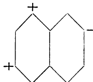
G Säure. D.R.P. 3229.
